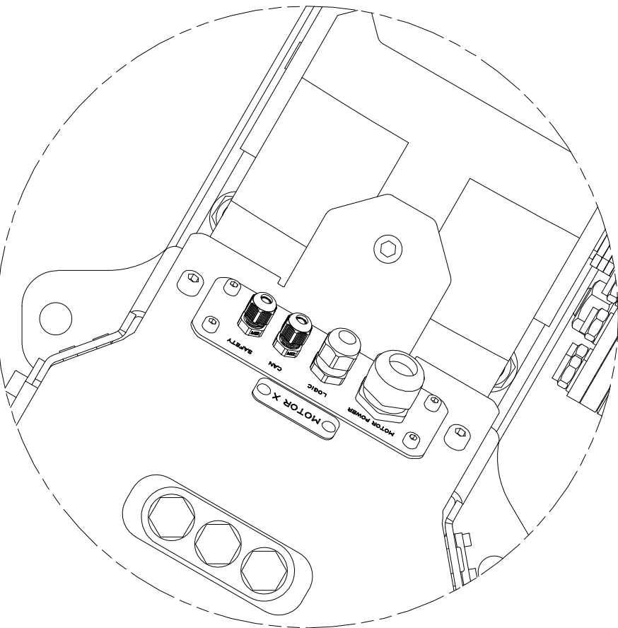
SZCZEGÓŁ C SKALA 1 / 3
